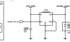
RCAM2 LDO
